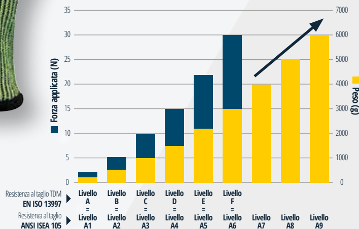
Equivalenza di taglio tra la norma europea e la norma ANSI*
