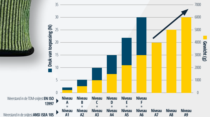
Equivalente eigenschappen tussen de Europese en de ANSI* normering.
