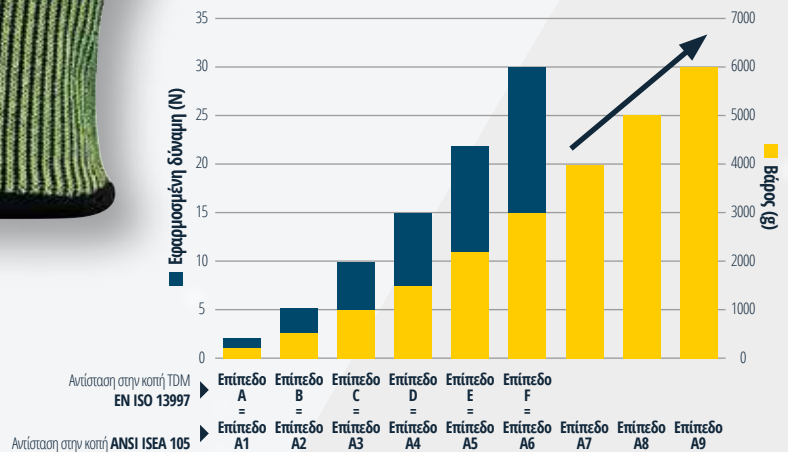
Ισοδυναμία της κοπής μεταξύ του ευρωπαϊκού προτύπου και του προτύπου ANSI*
